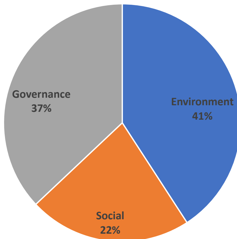
Grafico 2: Distribuzione dell'attività di engagement di tipo ESG per i comparti Bilanciato e Sviluppo
