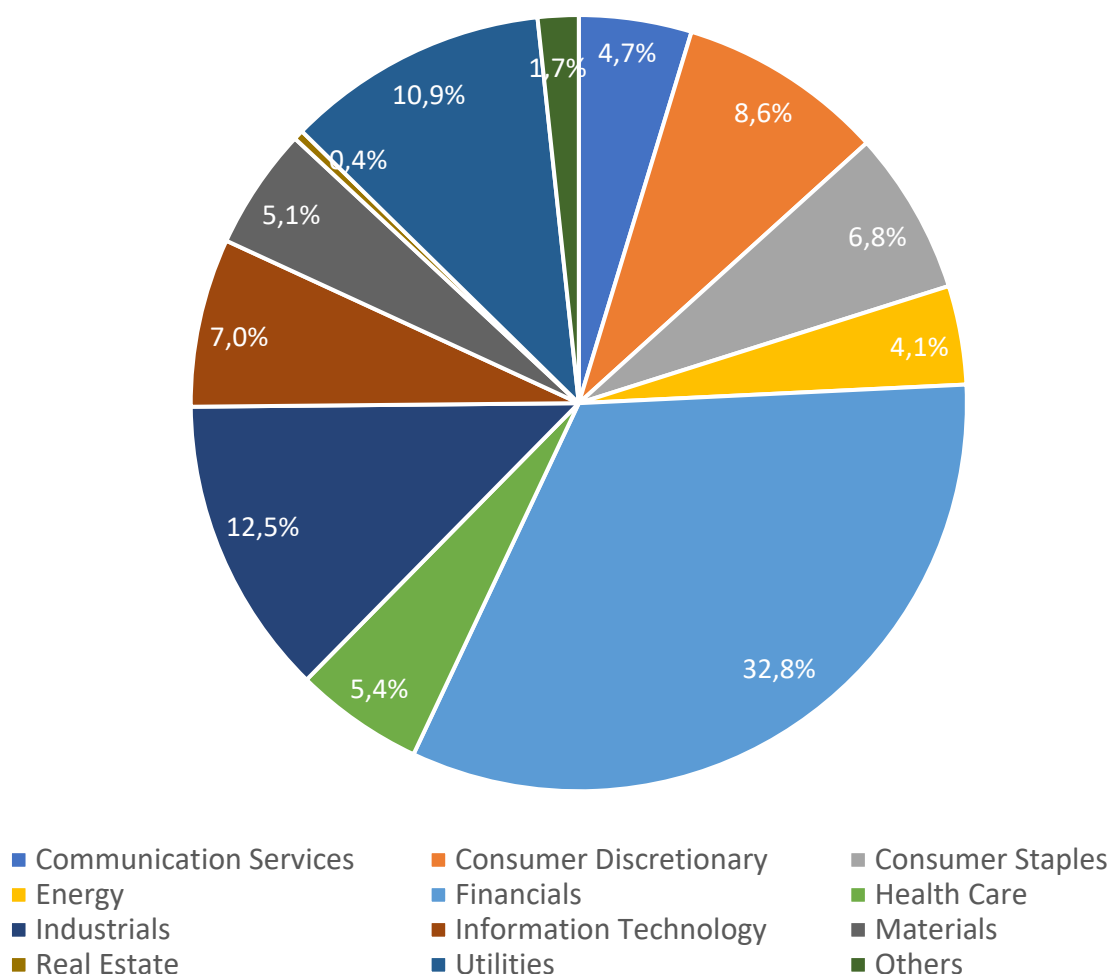
Grafico 1: Distribuzione per settori dell'attività di engagement per i comparti Bilanciato e Sviluppo
